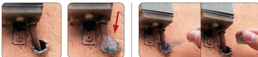
Protezione ingresso tubo corrugato
