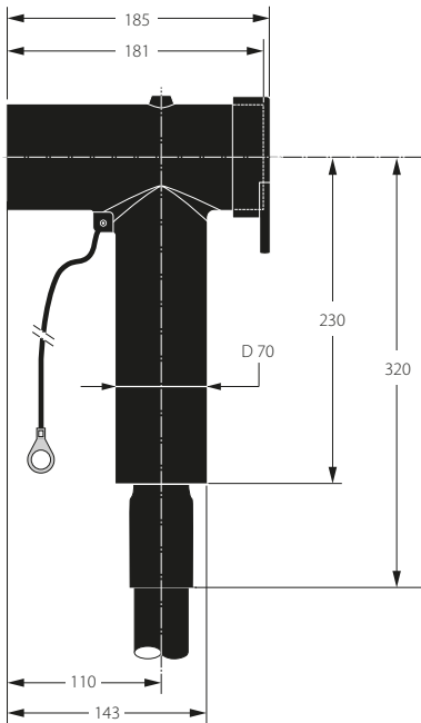
Kit de conexión Para cable apantallado con alambres incluido.
