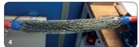
4 Metallabschirmung wieder herstellen
