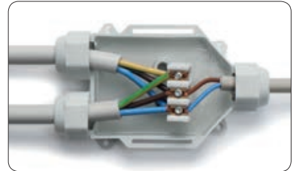
Mit integrierten Klemmenkasten.
